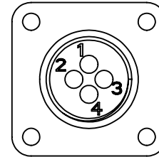
VIEW A-A
